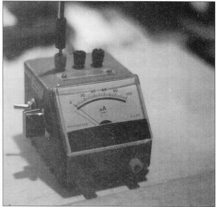
Boven: veldsterktemeter.
